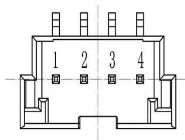
图10-3. 连接器
