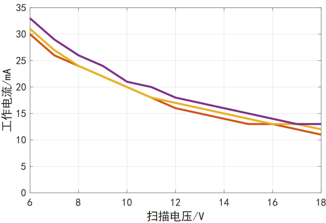
图7-3. 125℃工作电流曲线
