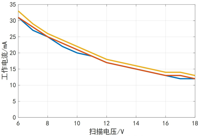
图7-1. -40℃工作电流曲线
