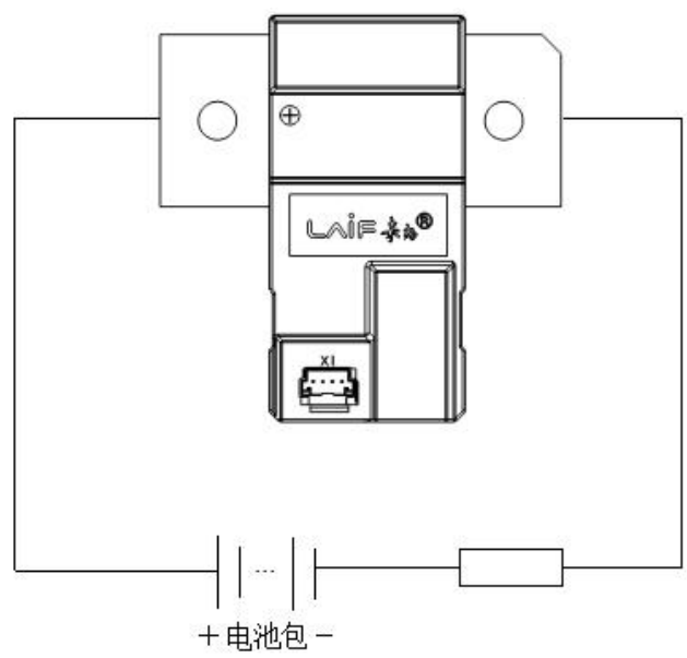
图9-1. 高压主正端推荐使用场景
