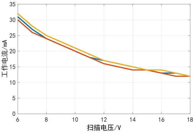
图7-2. 25℃工作电流曲线
