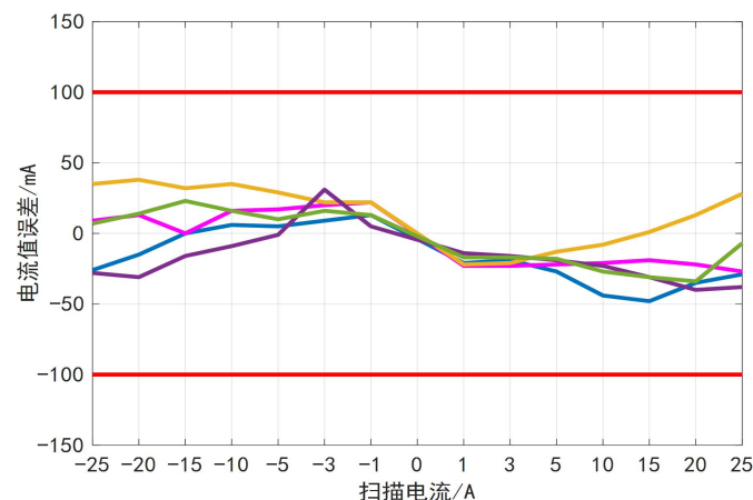
图7-6. 125℃小电流测试精度
