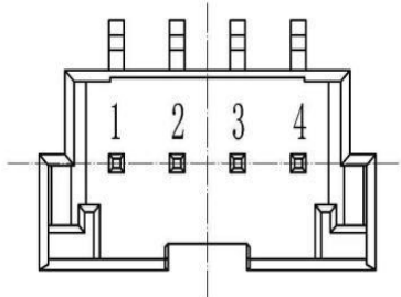
图10-3. 连接器
