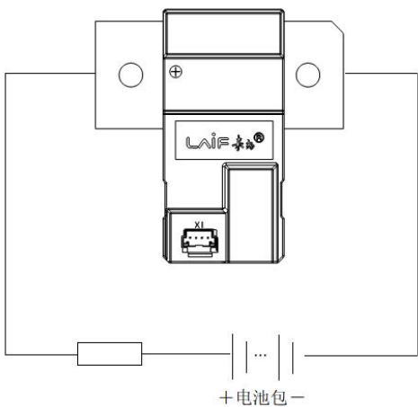
图 9. 高压主负端推荐使用场景
