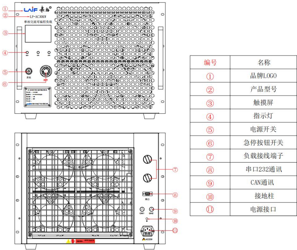
7-1 设备外观图-标准 8U
