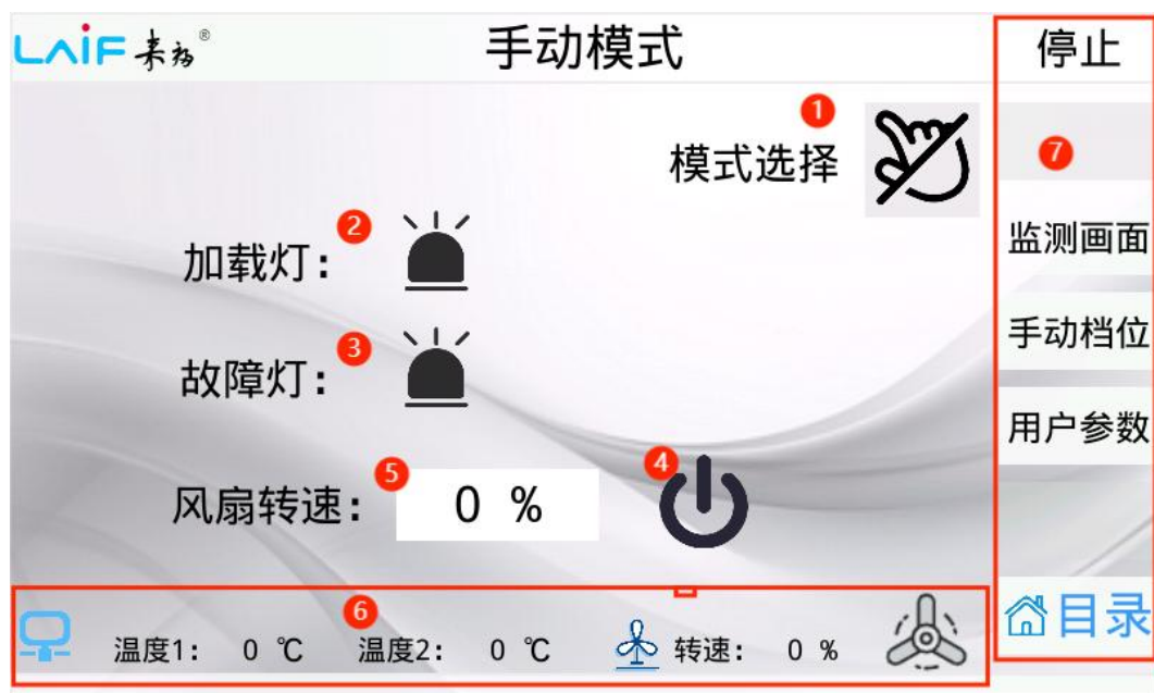
5-4 手动模式图
